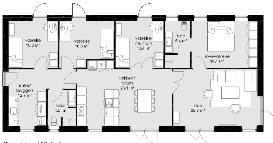
Grundplan 139,4 m 2
