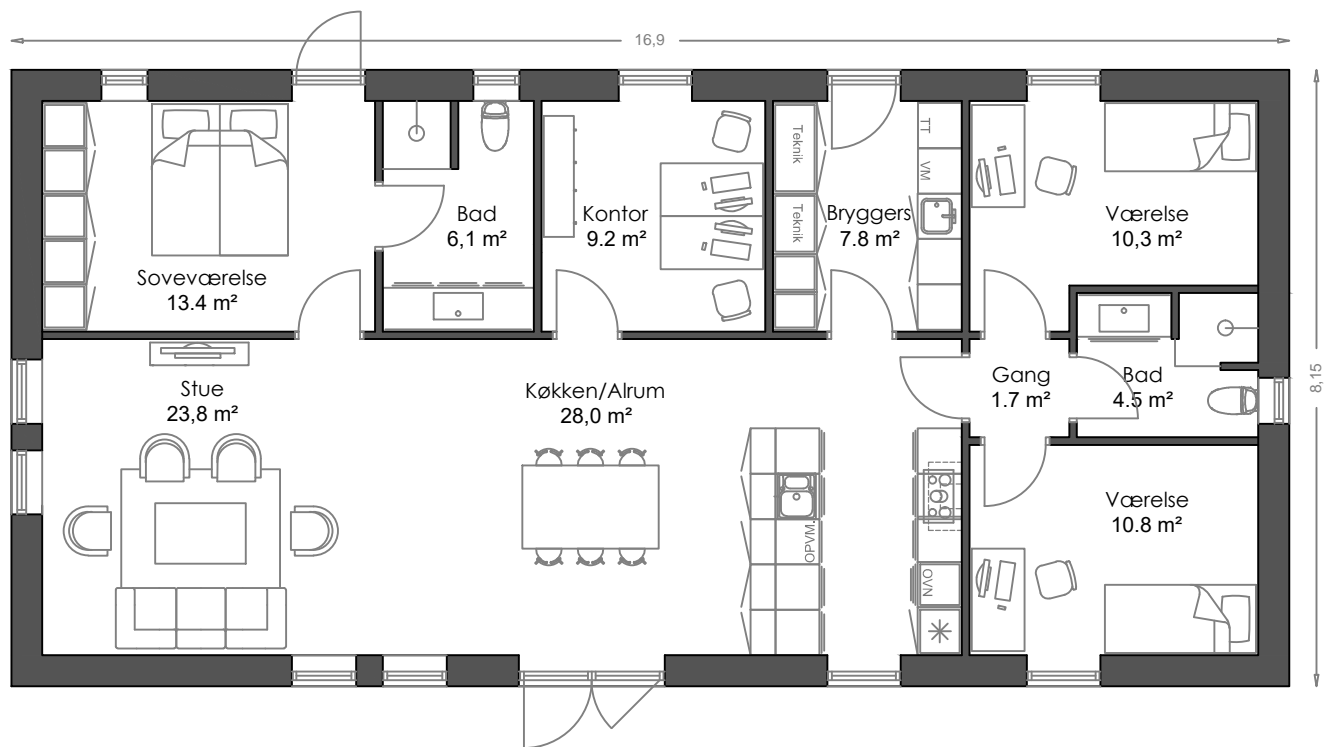
Grundplan 137,7 m²
