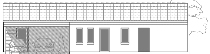
Facade nord
