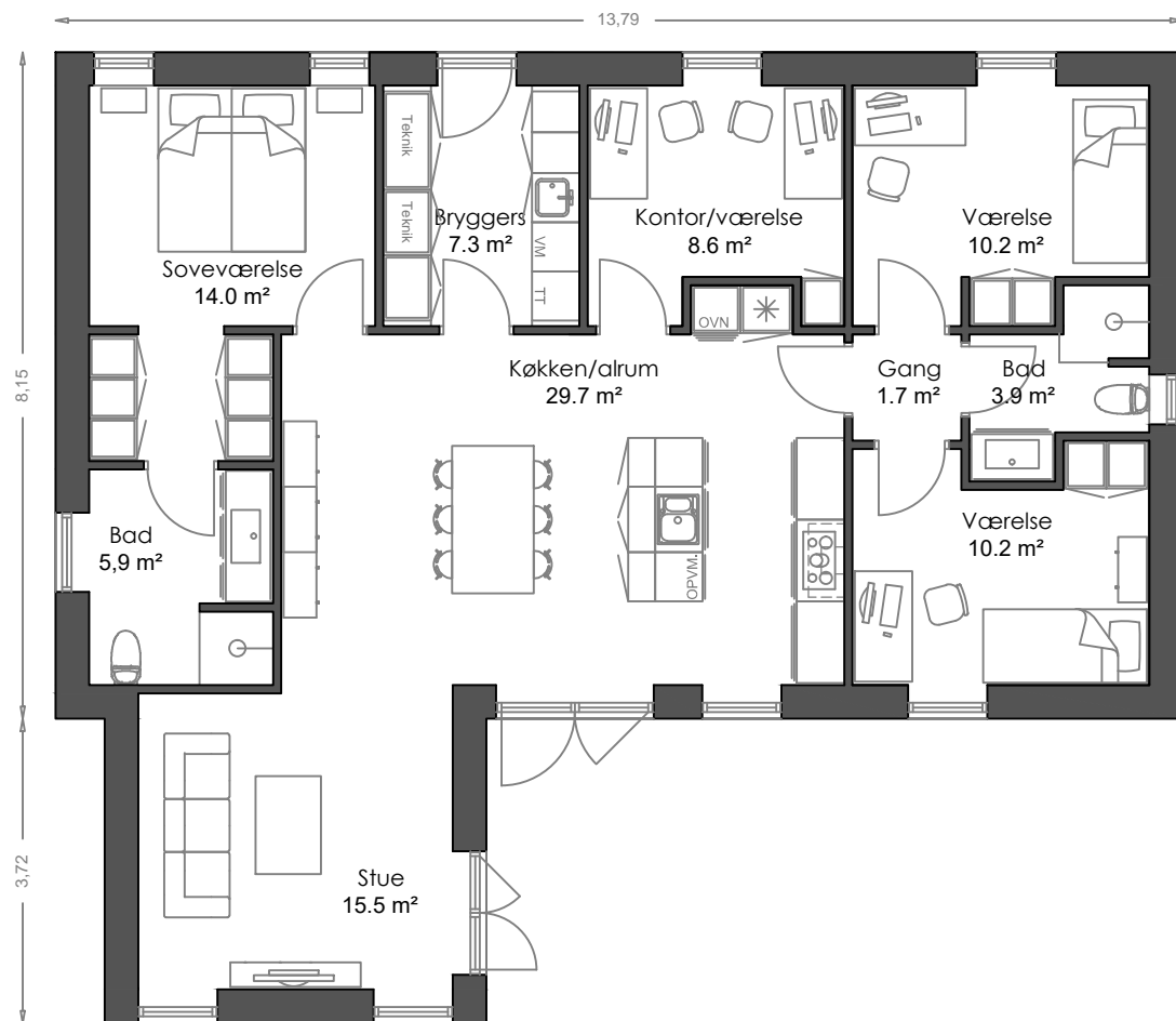
Grundplan 129.8 m 2 Indgang i facade
