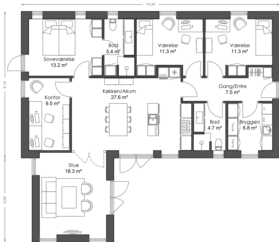
Grundplan 138.6 m 2 Indgang i Gavl
