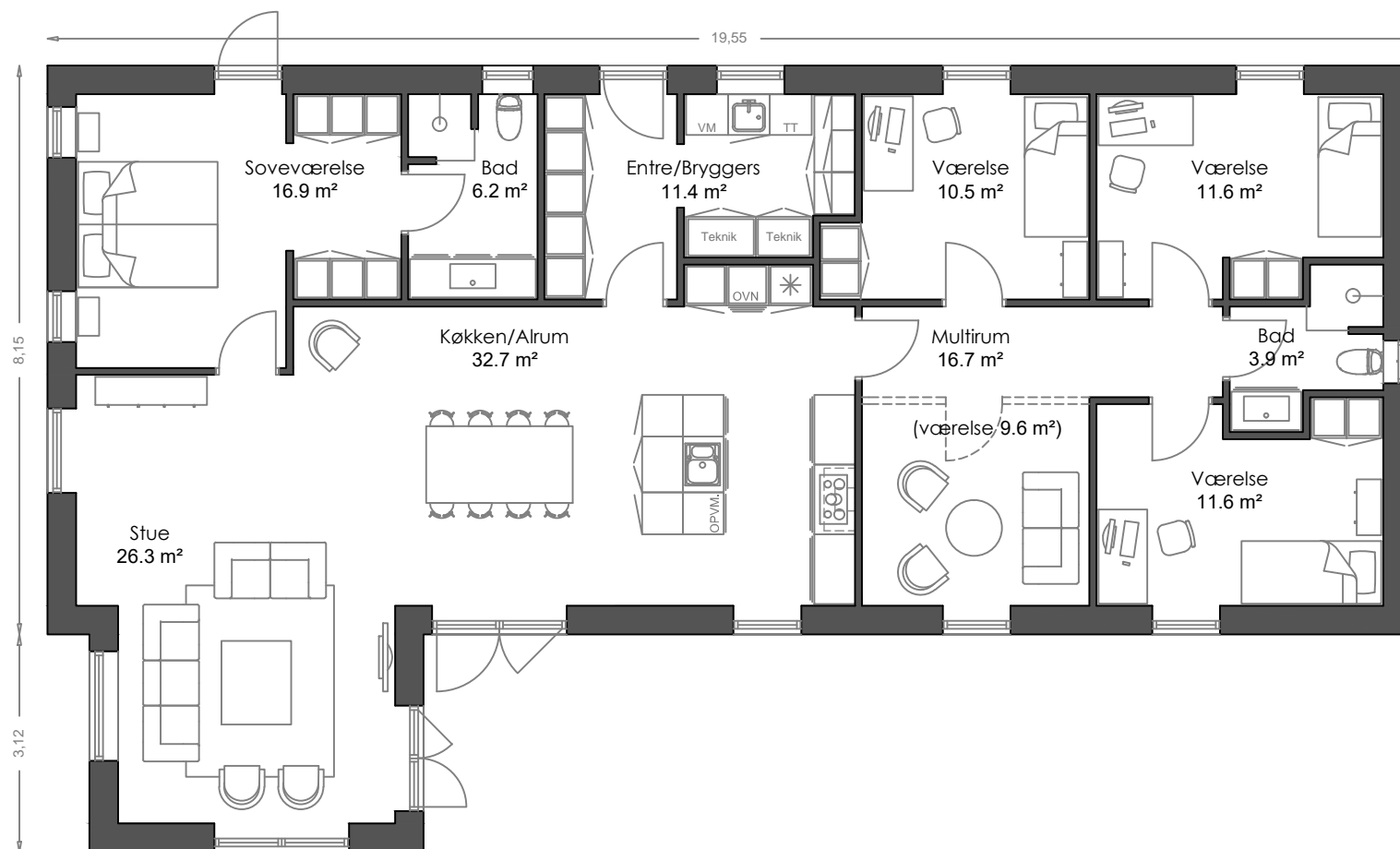
Grundplan 174.3 m 2 Indgang i facade
